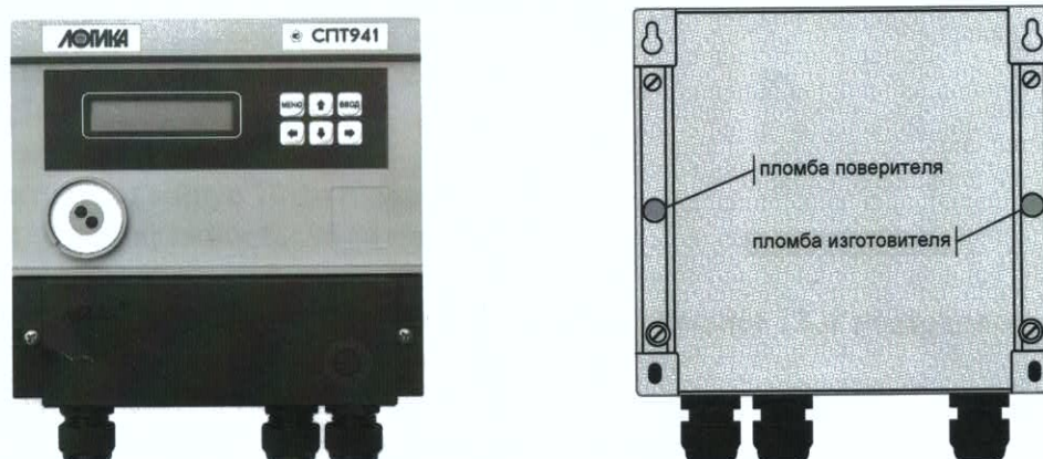
Рисунок 1 – Общий вид и схема пломбирования (вид сзади)
